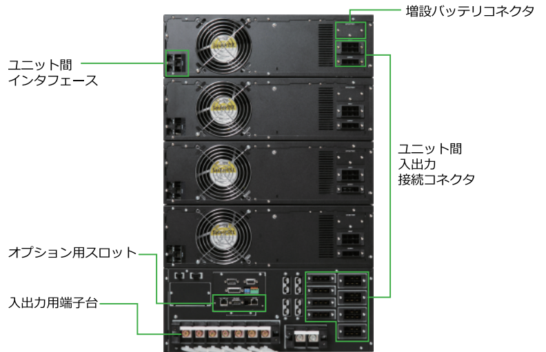
《UPSS-200X2-005RM/5 背面》
