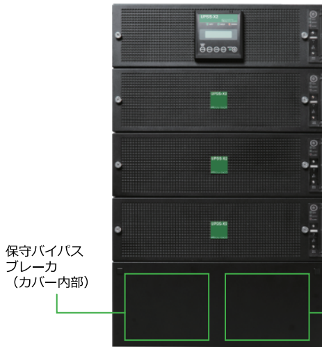
《UPSS-200X2-005RM/5 正面》
