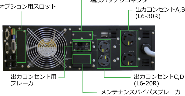
《UPSS-200X2-005RM/5 背面》
