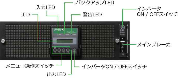
《UPSS-50X2-005RMC/5 正面》
