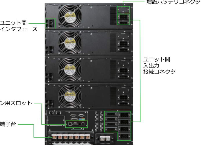
《UPSS-200X2-005RM/5 背面》
