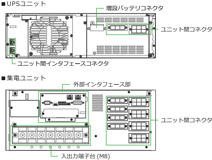
《UPSS-200X3-005RM/5 背面》
