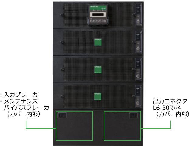
《UPSS-200X3-005RM/5 正面》
