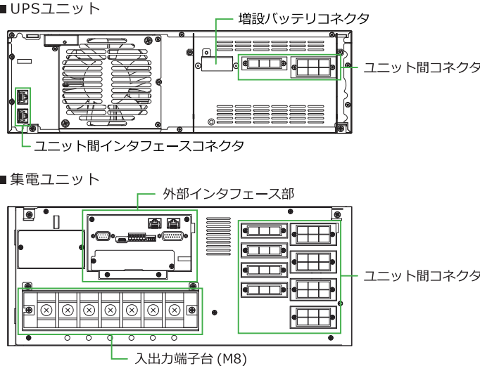
《UPSS-200X3-005RM/5 背面》
