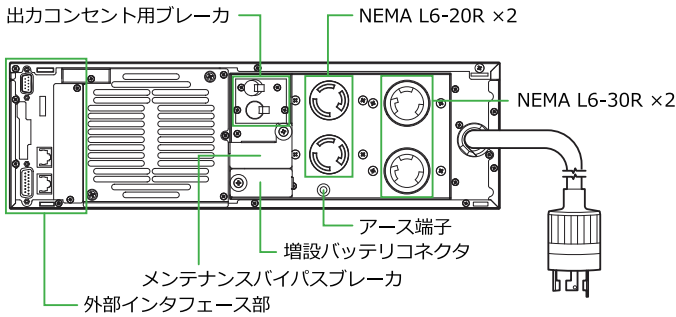
《UPSS-200X3-005RM/5 背面》
