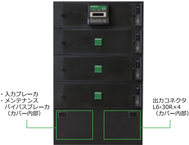
《UPSS-200X3-005RM/5 正面》
