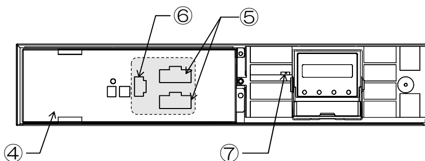
バッテリー押さえ金具の内側
