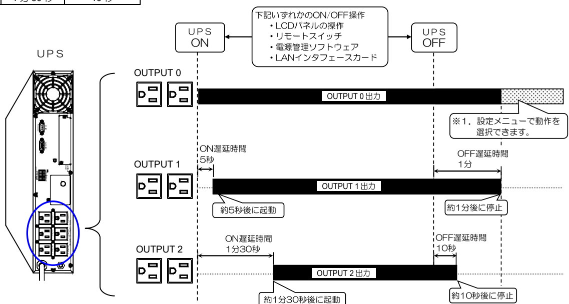
系統コントロールによる OUTPUT0, 1, 2 の出力状態
