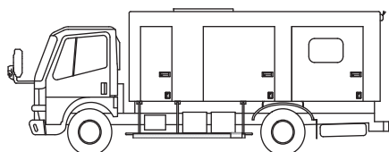
■ 3.5t 車 100kW GENERATOR サイズ：L6,350×W2,120×H2,440mm 重量：6,760Kg
