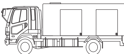
■ 4t 車 300kW GENERATOR サイズ：L6,990×W2,270×H2,680mm 重量：7,820Kg
