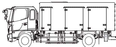
■ 8t 車 100kW GENERATOR ×2 台積み サイズ：L7,300×W2,360×H2,730mm 重量：10,150Kg
