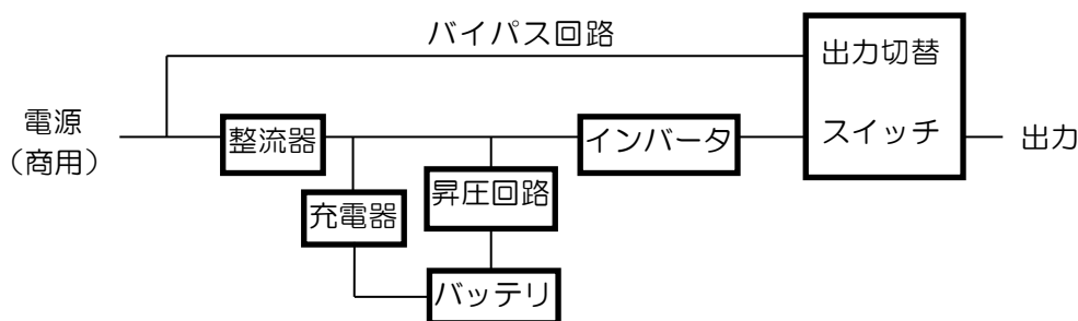
過負荷停止時の電力供給経路
