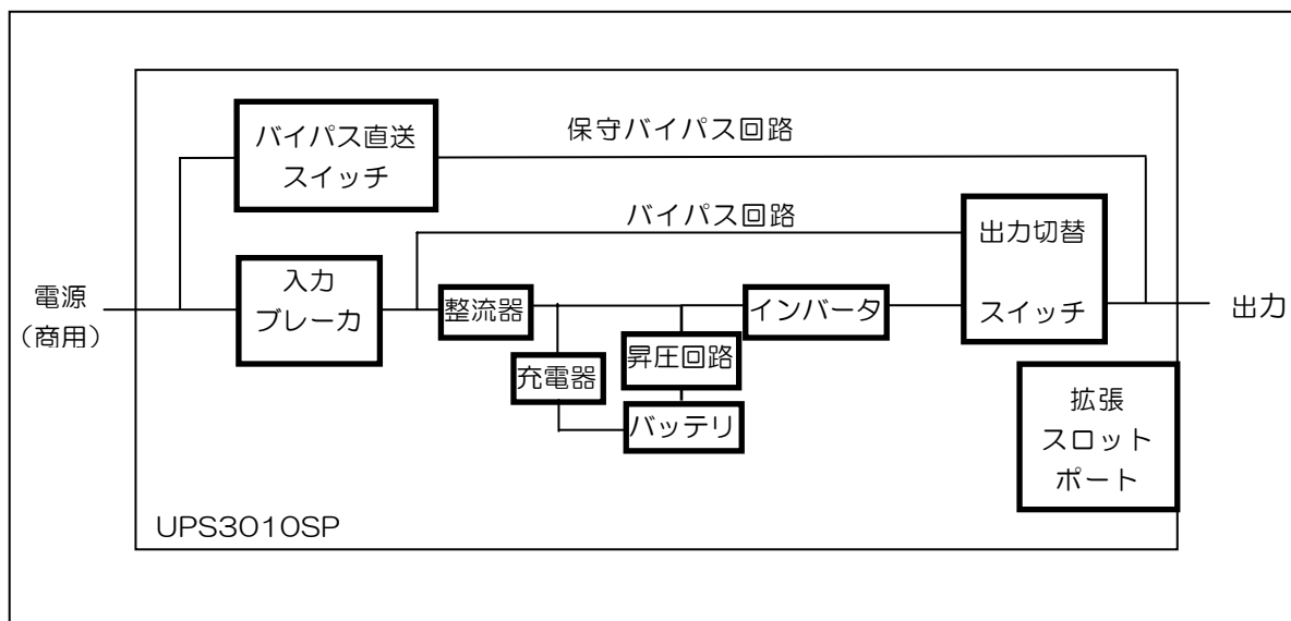
UPS3010SP 概略構成図
