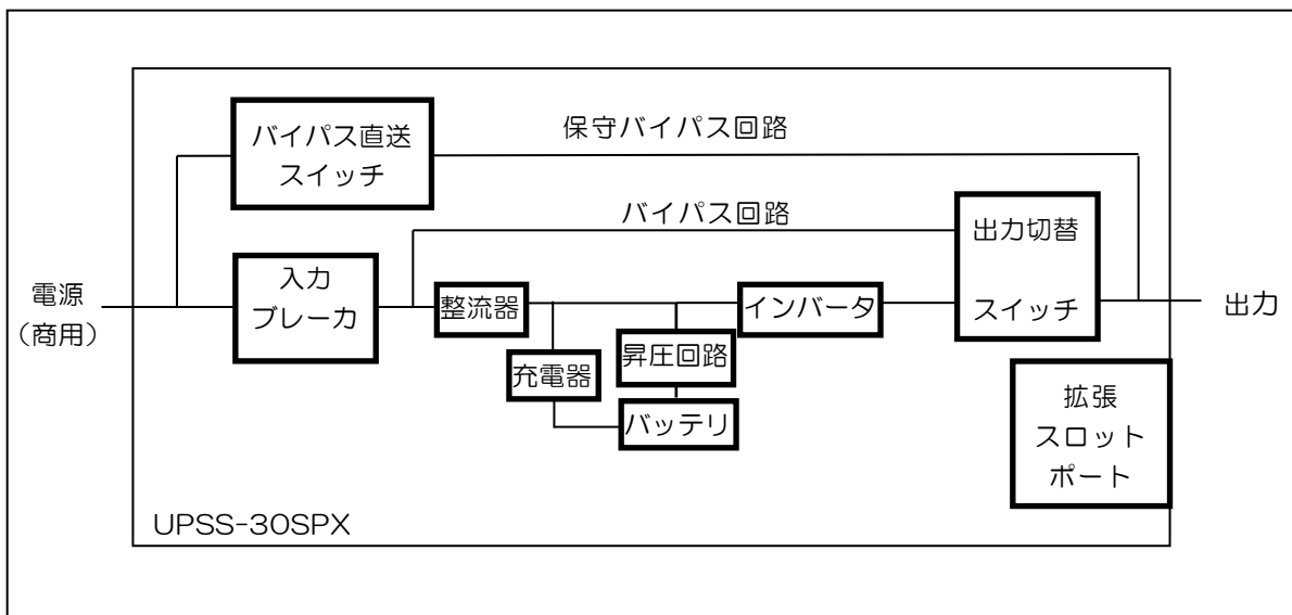
UPSS-30SPX 概略構成図
