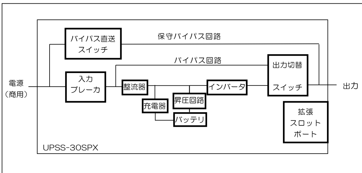
UPSS-30SPX 概略構成図
