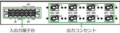
UPSS-ITRD-3.5K2UIR (3.5kVA)
