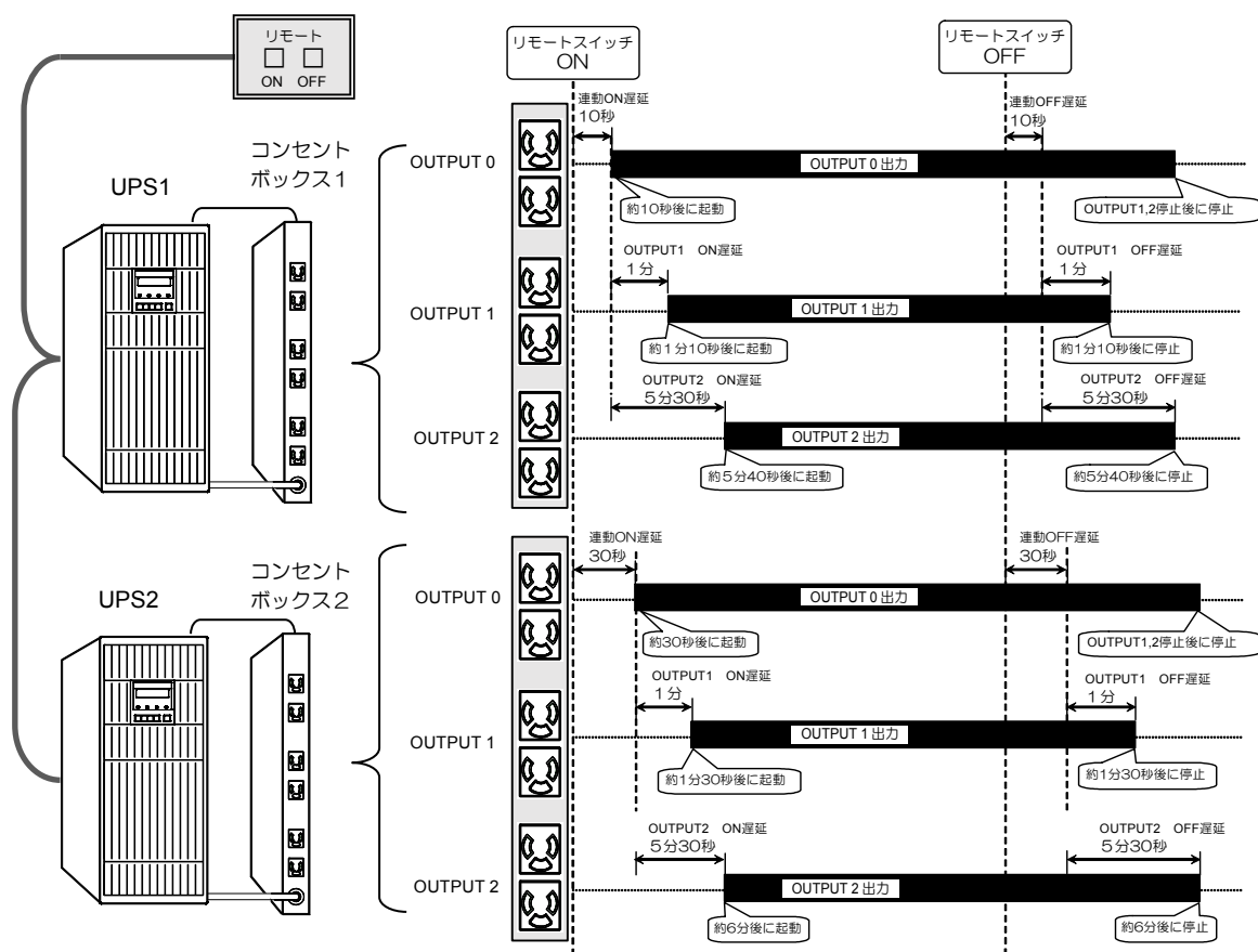
系統コントロールと連動運転を併用した場合の出力状態
