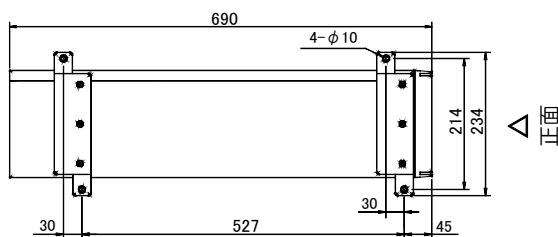
床固定寸法
