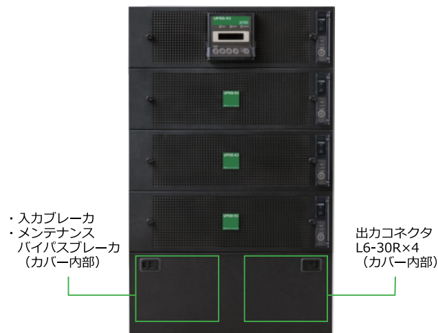
《UPSS-200X3-005RM/5 正面》
