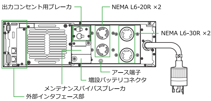
《UPSS-50X3LI-010RMC 背面》
