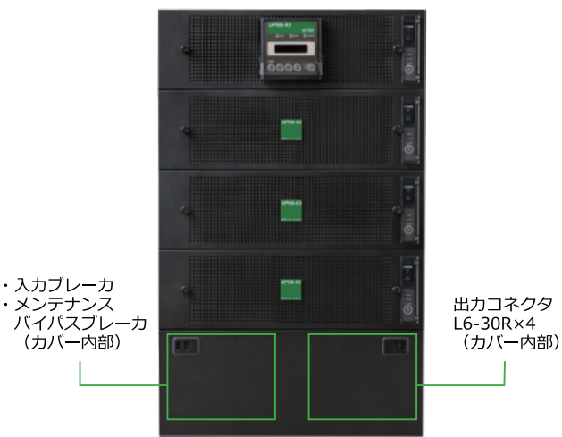
《UPSS-200X3LI-010RM 正面》
