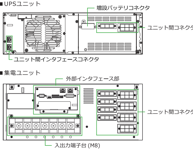
《UPSS-200X3LI-010RM 背面》
