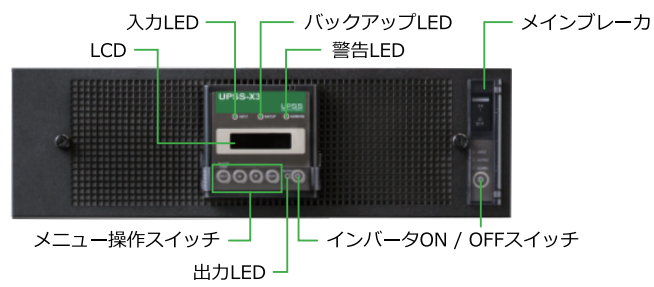
《UPSS-50X3LI-010RMC 正面》
